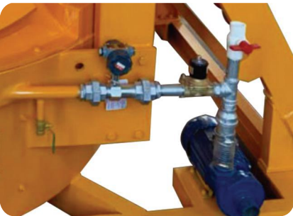
水泵&流量计量系统 Pump & Flow Metering System
